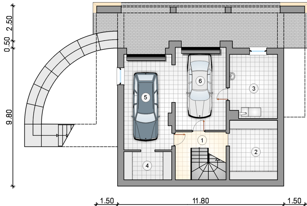
RZUT PIWNICY
