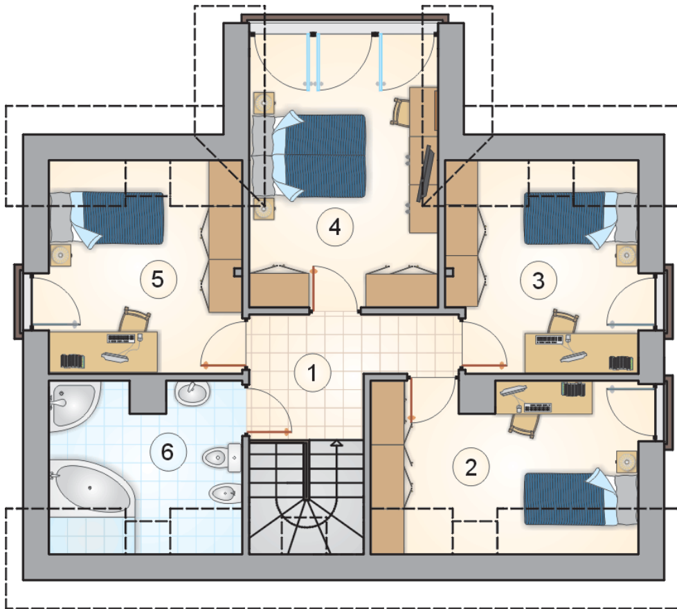
RZUT PODDASZA
