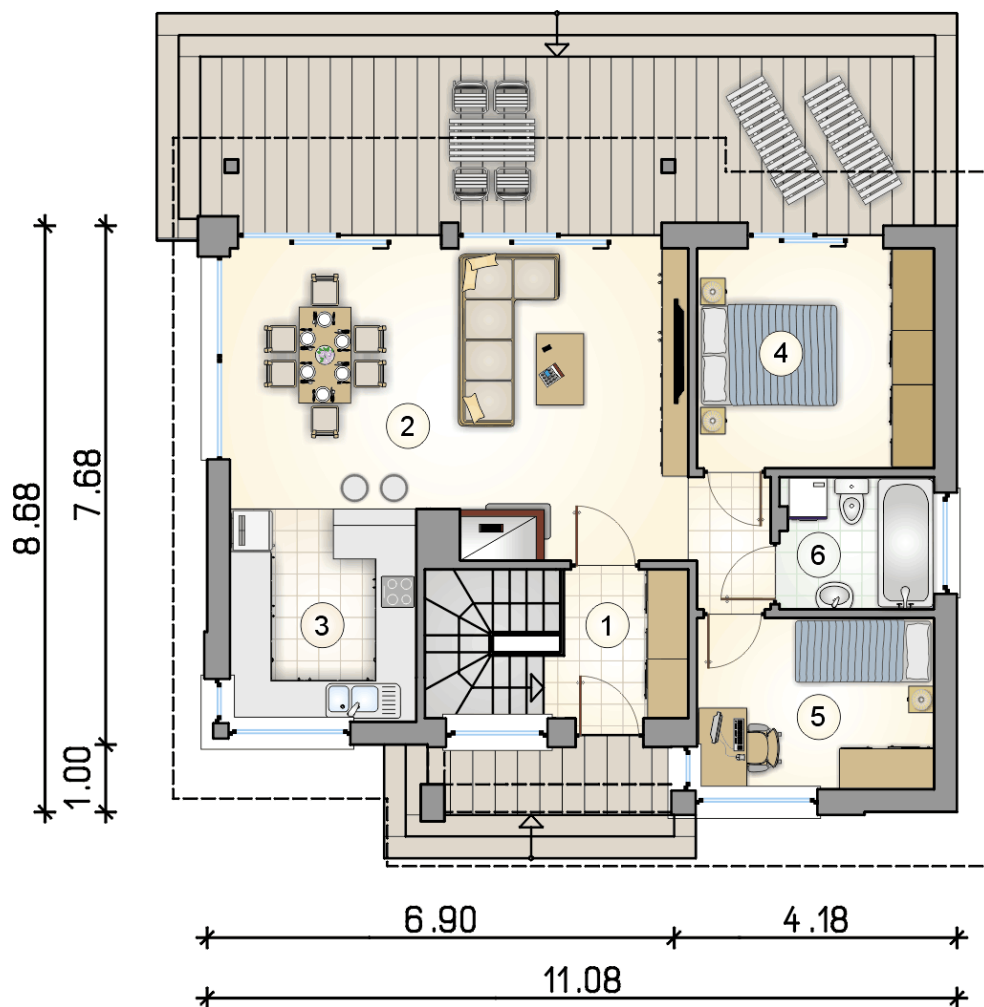
RZUT PARTERU
