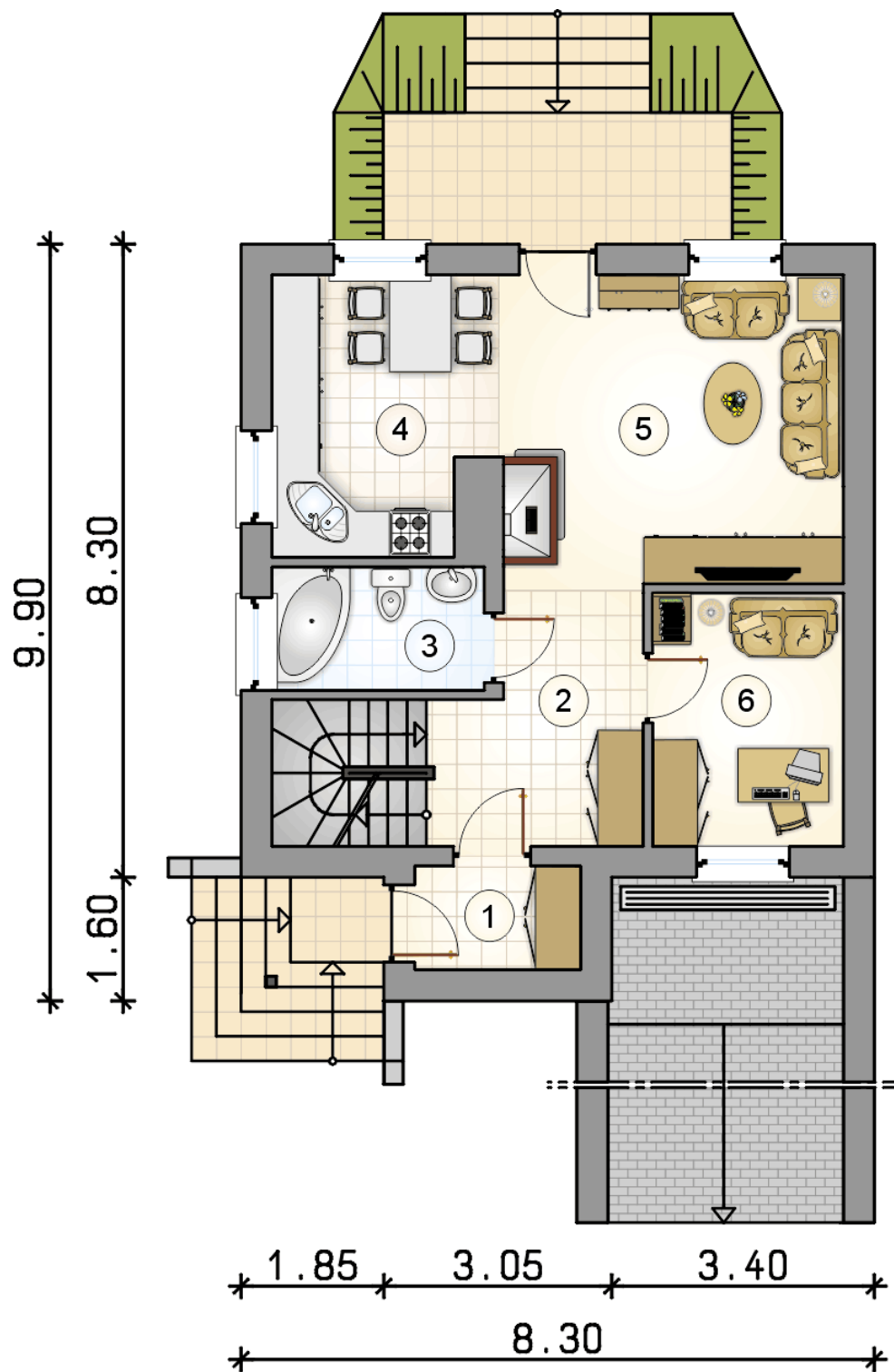
RZUT PARTERU
