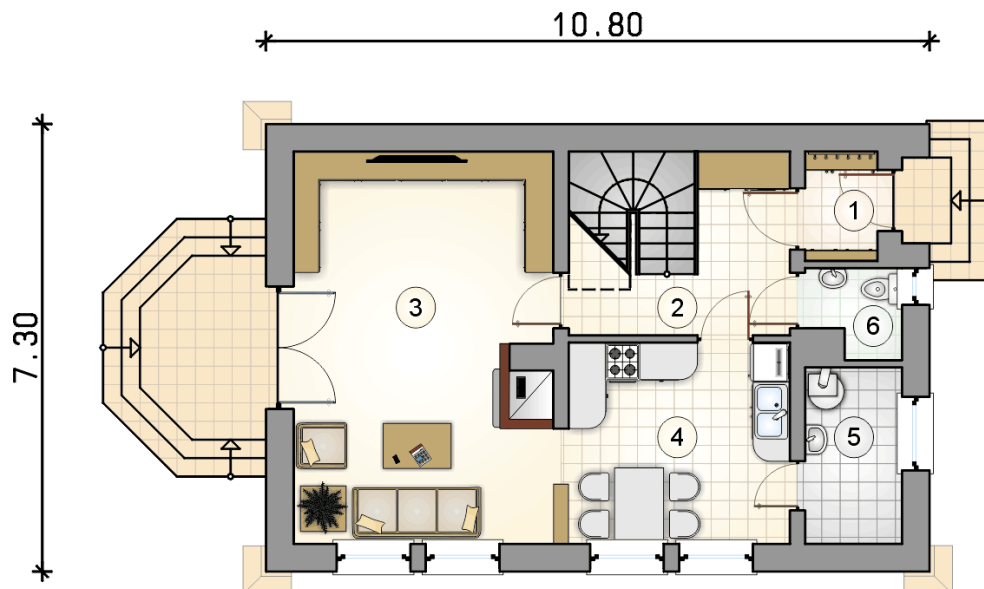
RZUT PARTERU
