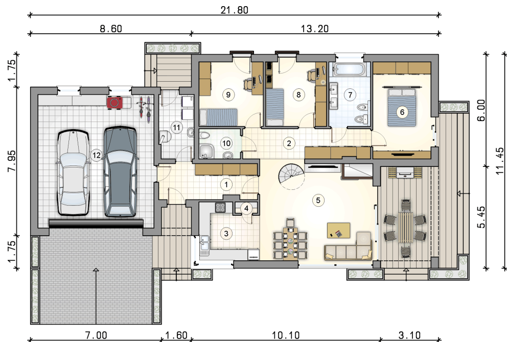
RZUT PARTERU PROJEKTU KOS VIII
