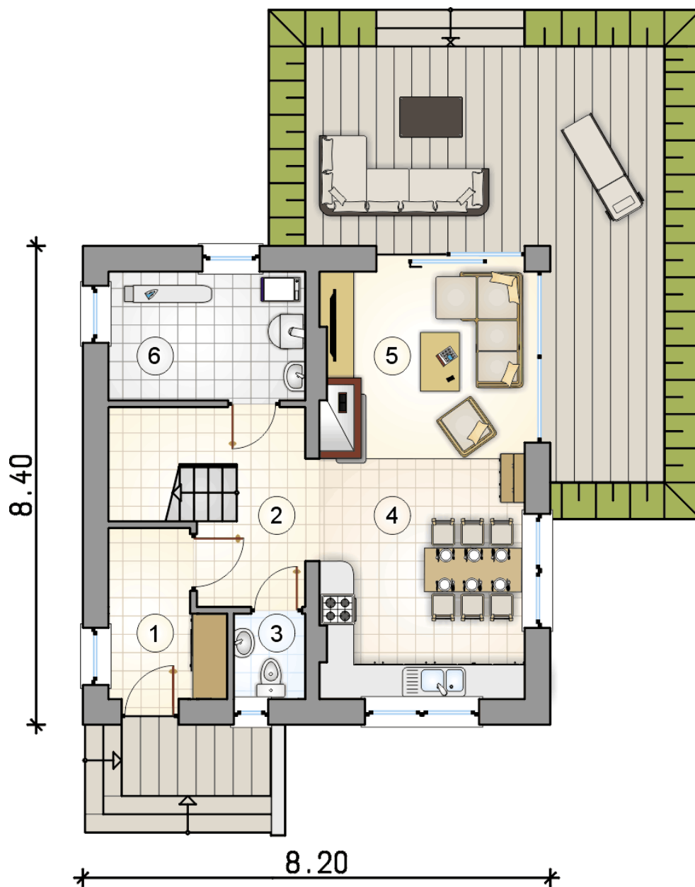
RZUT PARTERU
