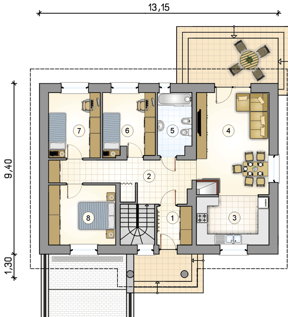
RZUT PARTERU
