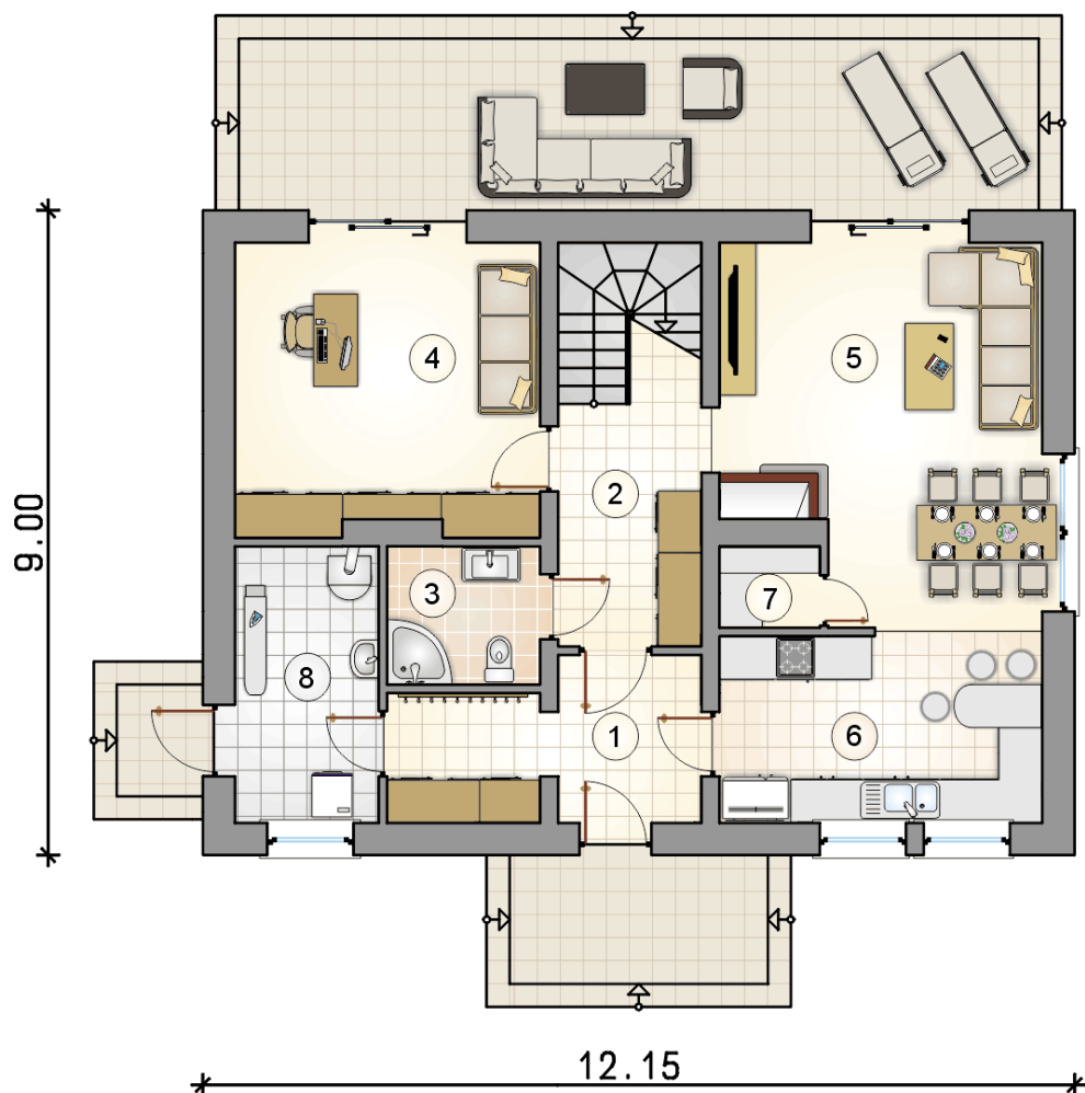
RZUT PARTERU
