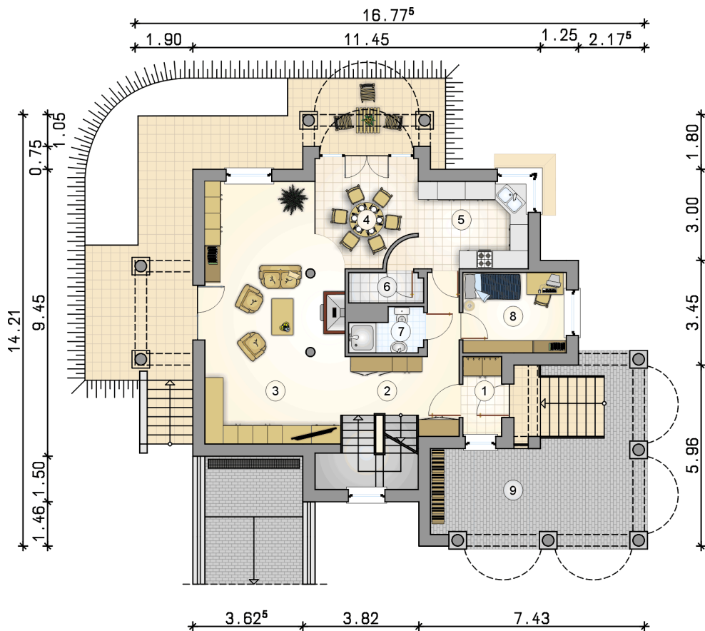
RZUT PARTERU
