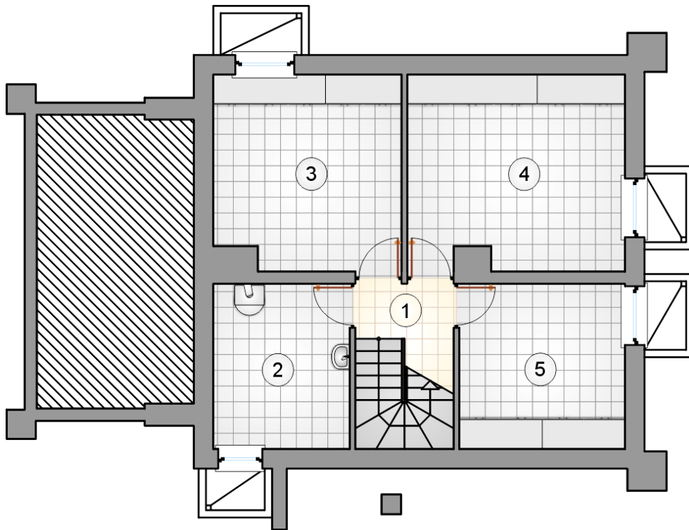
RZUT PIWNICY
